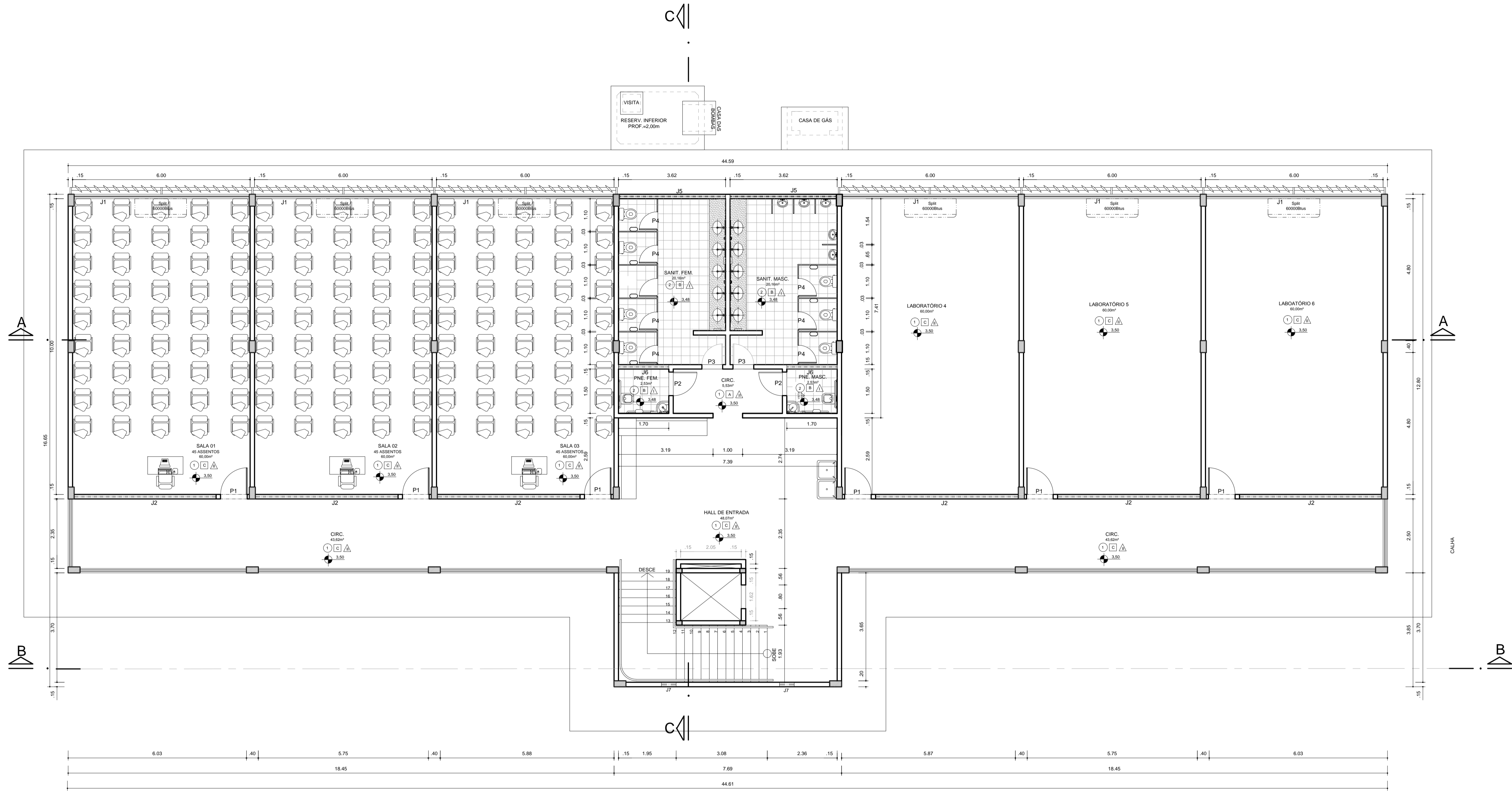
PLANTA BAIXA - 1º PAVIMENTO ESC. 1/75
